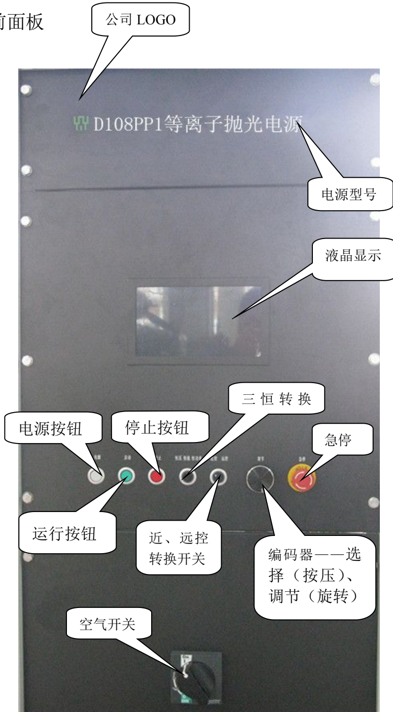
电源前面板示意图（图一）
