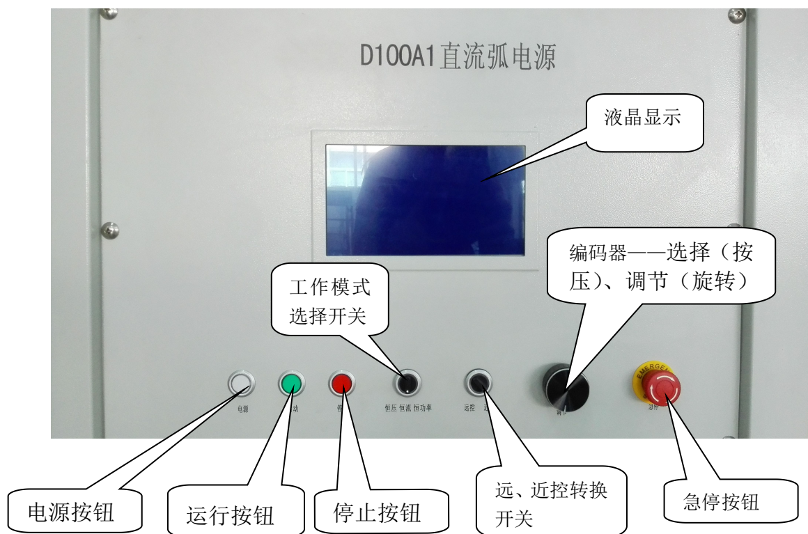
电源前面板示意图（图一）
