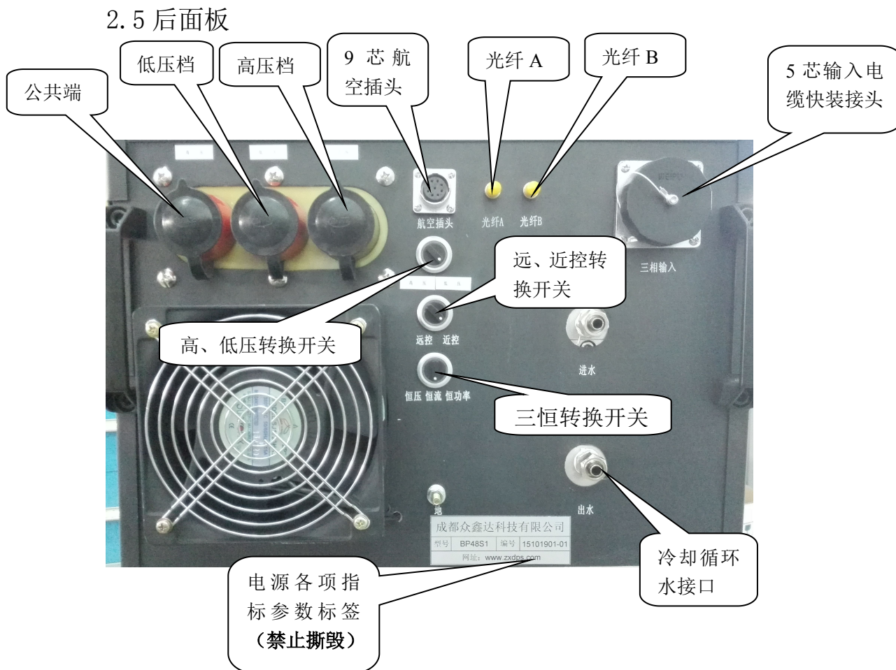
电源后面板示意图 (图二)
