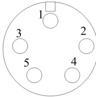
WS48-5P 1:接地 2 4 5:三相380VAC±5% 3:零线 电缆线径推荐值: 36KW:16平方毫米 地线: 6平方毫米
