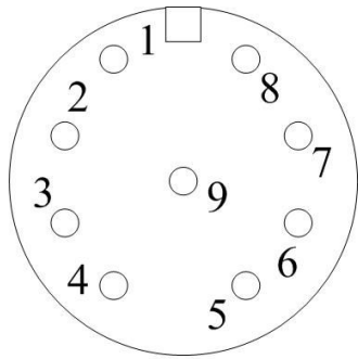
WS20-9P 1 2:水流电磁阀开关 3 4:电源运行状态无源触点 8 9:门锁保护(已短接) 5 6 7:备用
