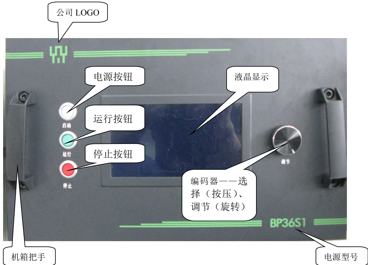
电源前面板示意图（图一）
