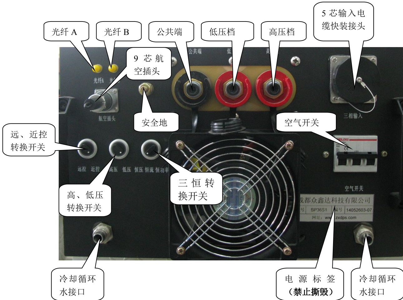
电源后面板示意图（图二）
