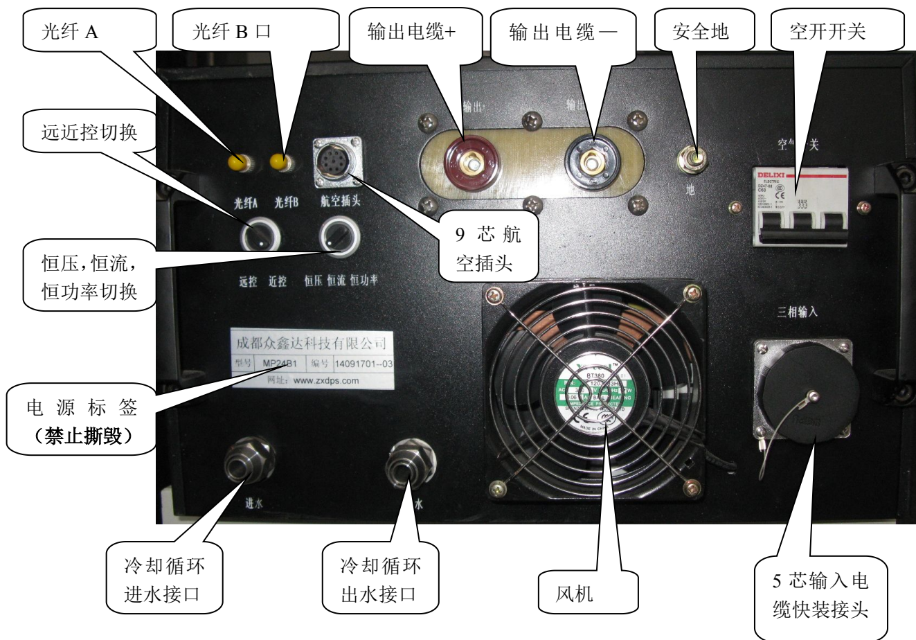
电源后面板示意图 (图二)
