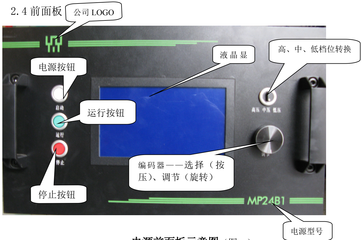
电源前面板示意图（图一）
