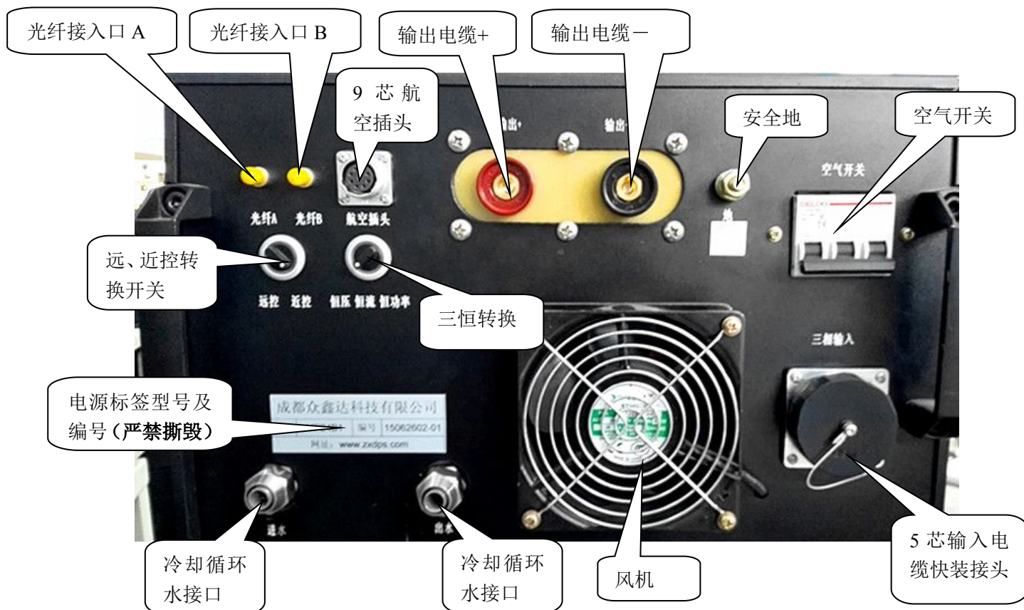
电源后面板示意图 (图二)
