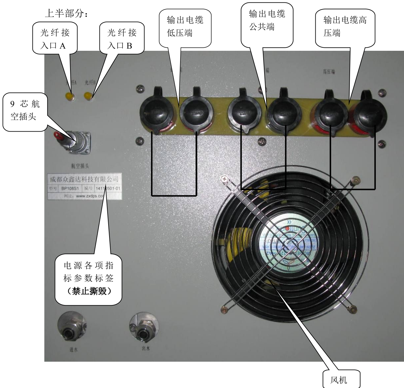
电源后面板示意图 (图三)
