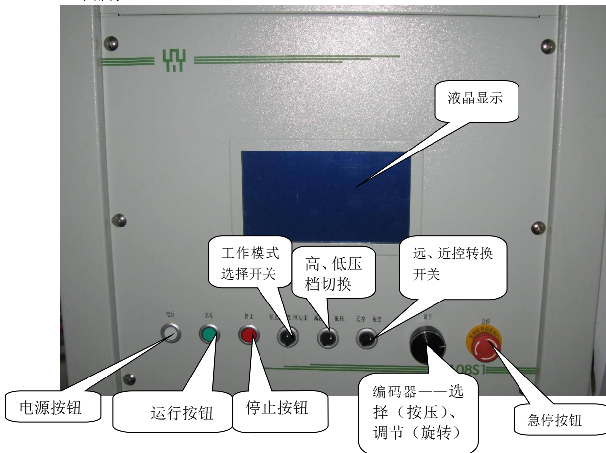
电源前面板示意图（图一）
